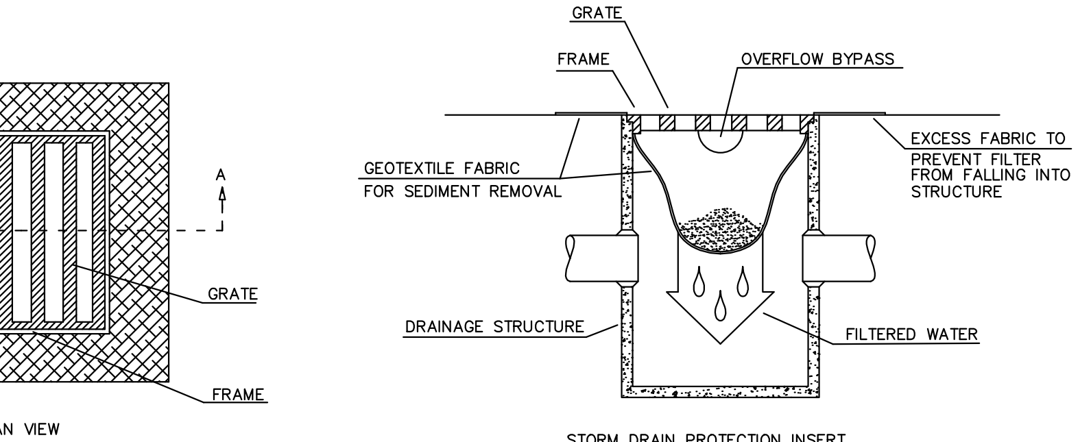
STORM DRAIN PROTECTION INSERT SECTION A-A N.T.S.
